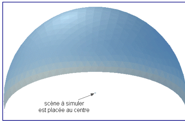
figure B.1.2 : éclairements du ciel obtenus avec 6S formant la voûte céleste dans un raytracer
