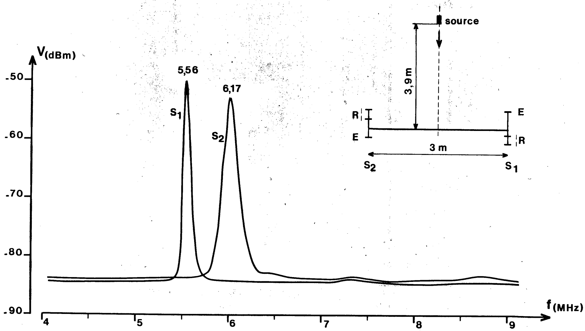
Fig.7 Réponses dans le plasma des sondes isoprobes fonctionnant simultanément
