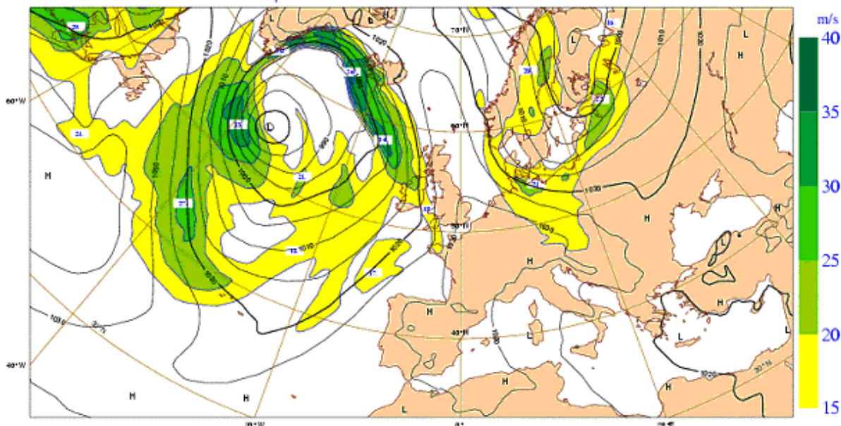
Figure 14 : Exemple de sortie du modèle numérique de prévision du climat ECMWF ( http://www.ecmwf.int/ )
