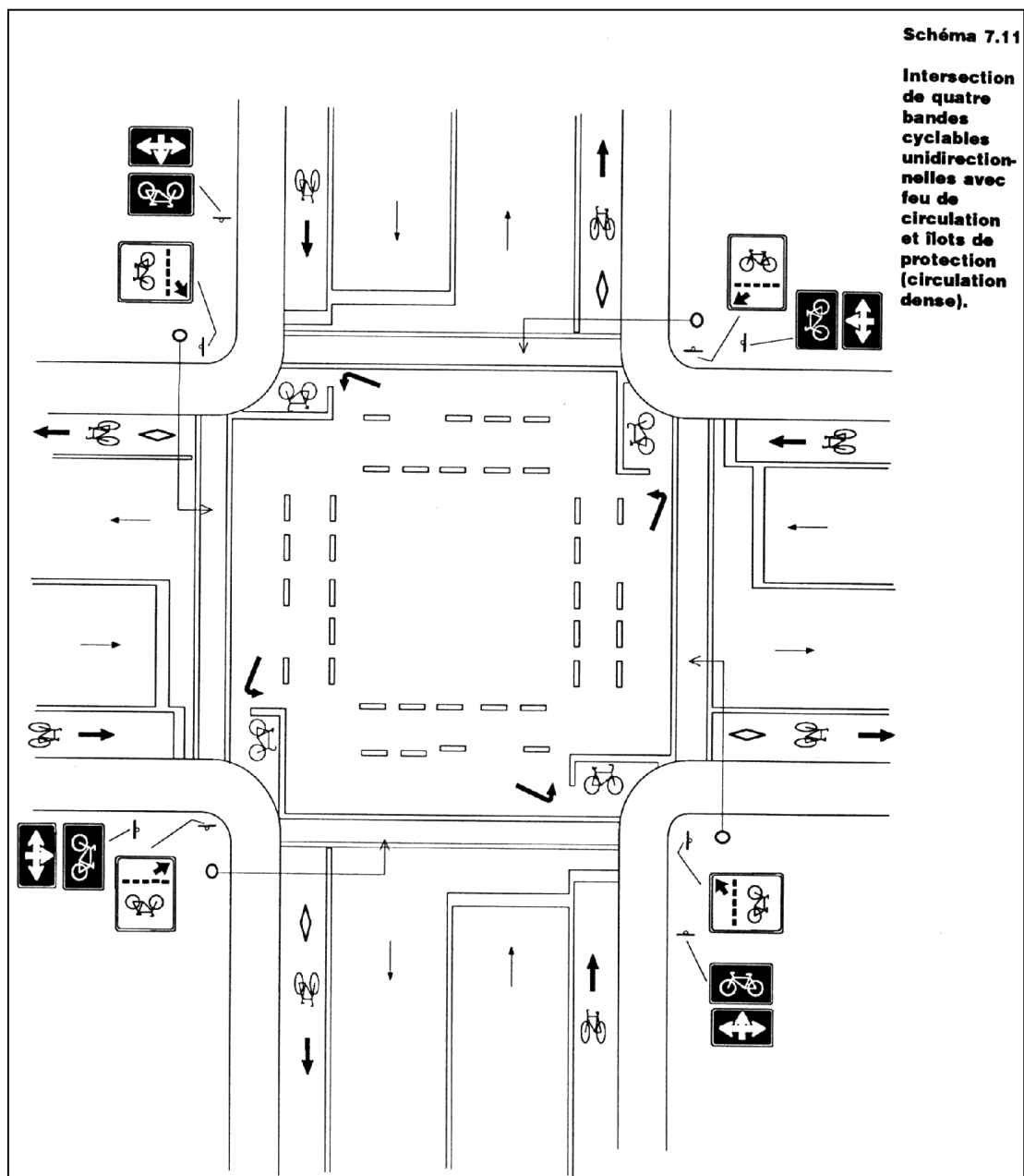
Figure 15 : Tourne-à-gauche indirect (Québec)
