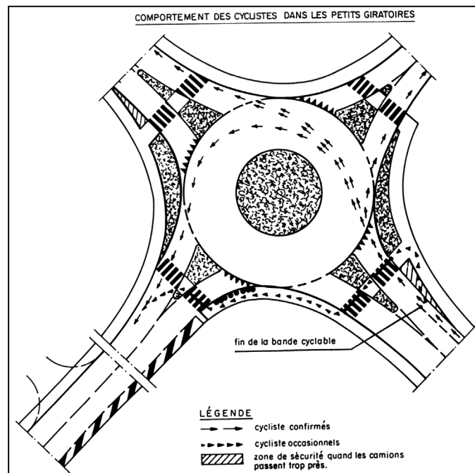
Figure 19 : Mini-giratoire (Suisse)
