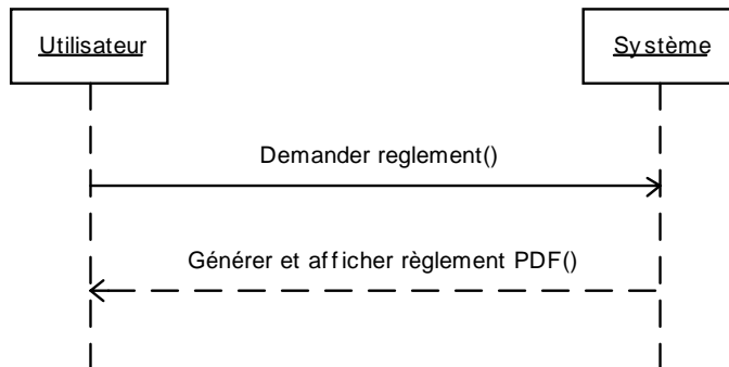
Figure 14 : Séquence d'opération correspondant à la génération du règlement au format PDF
