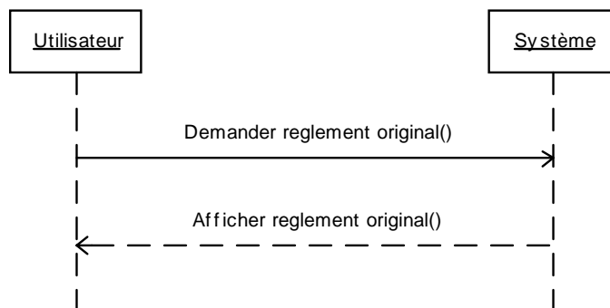
Figure 16 : Séquence d'opérations permettant de consulter le document original du règlement
