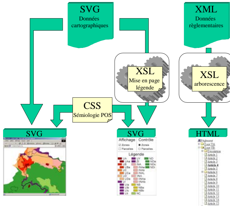
Figure 24 : Utilisation de CSS et XSL dans la maquette
