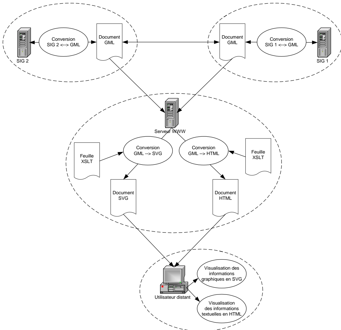
Figure 41 : Architecture préconisée pour l'échange et la consultation de données géographiques
