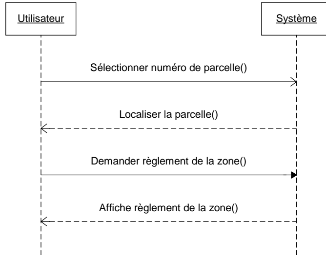
Figure 12 : Séquence d'opérations correspondant à la localisation d'une parcelle et à l'affichage du règlement de la zone correspondante
