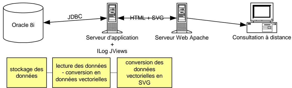
Figure 42 : Architecture proposée avec ILog JViews
