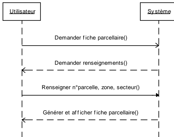
Figure 13 : Séquence d'opérations correspondant à la génération d'une fiche parcellaire
