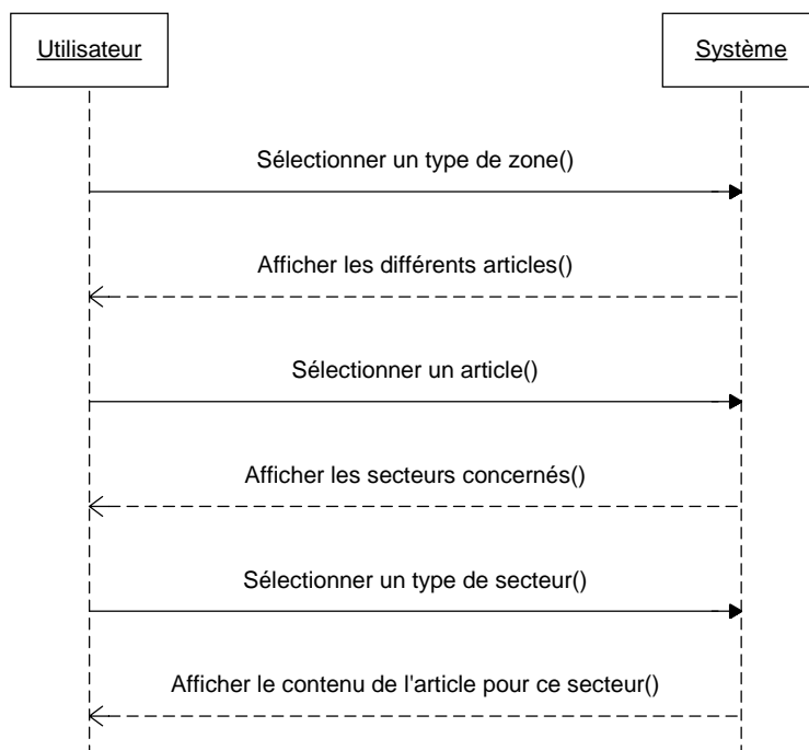
Figure 11 : Séquence d'opérations pour visualiser le règlement pour un type de zone et/ou un type de secteur
