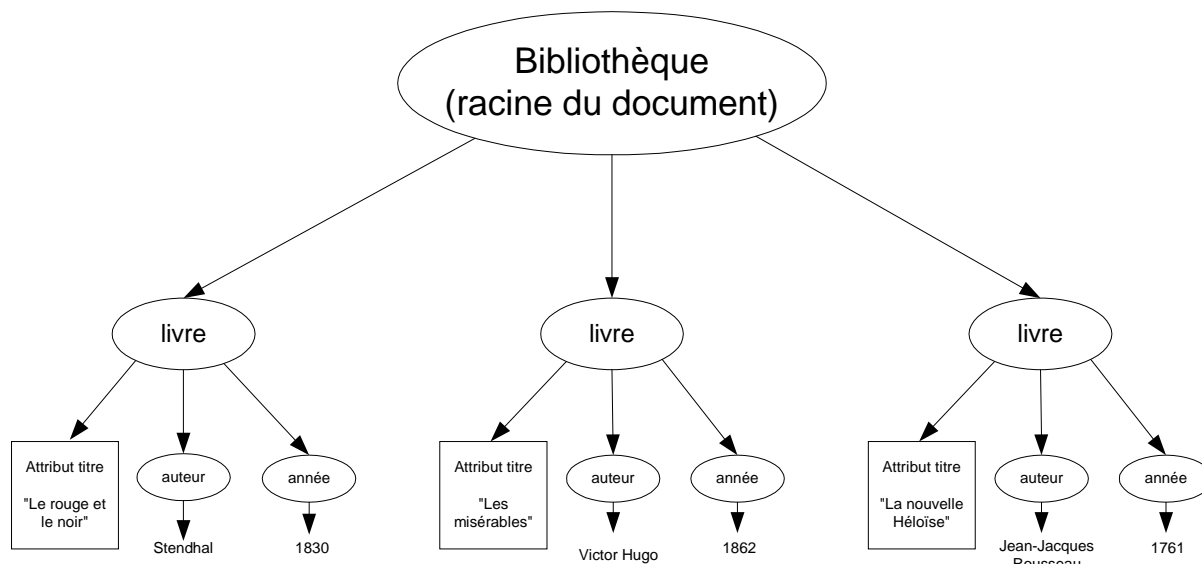
Figure 17 : Hiérarchie d'un document XML
