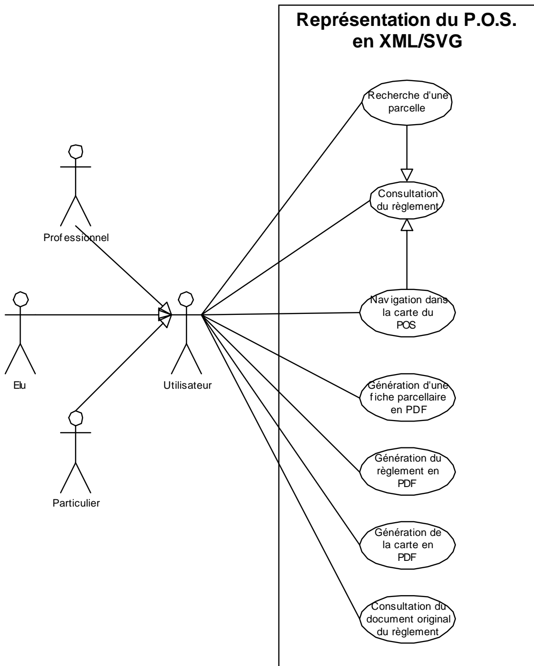
Figure 9 : Les différents cas d'utilisation
