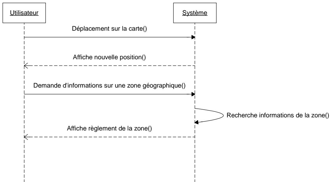
Figure 10 : Séquence d'opérations correspondant à la localisation d'une zone géographique et l'affichage de son règlement
