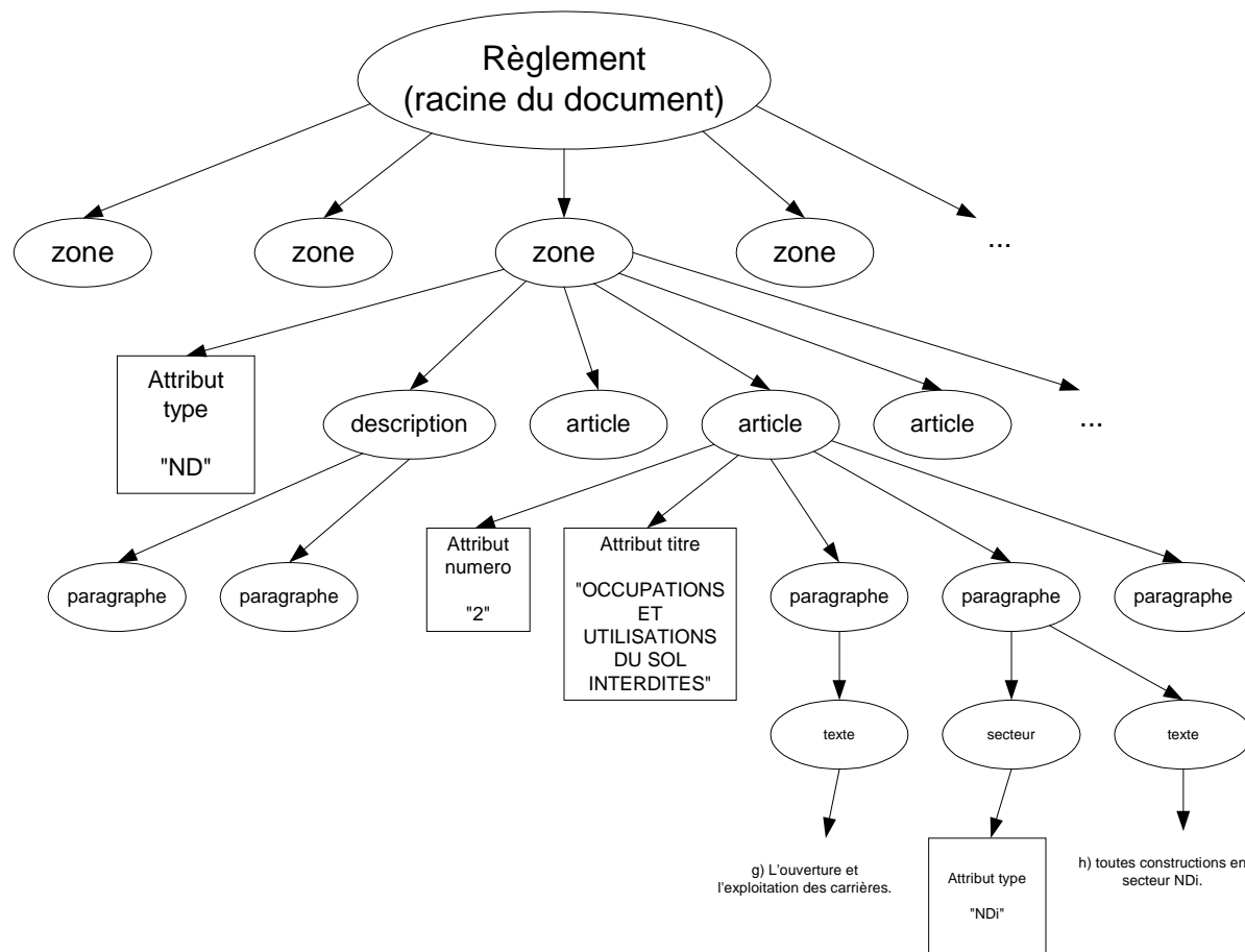
Figure 18 : Hiérarchie du document du règlement
