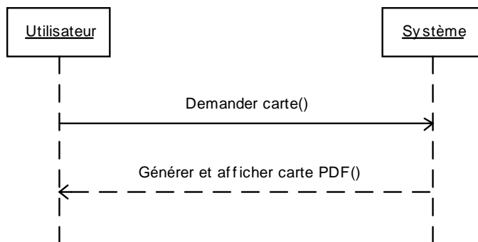
Figure 15 : Séquence d'opérations correspondant à la génération de la carte du P.O.S. au format A3
