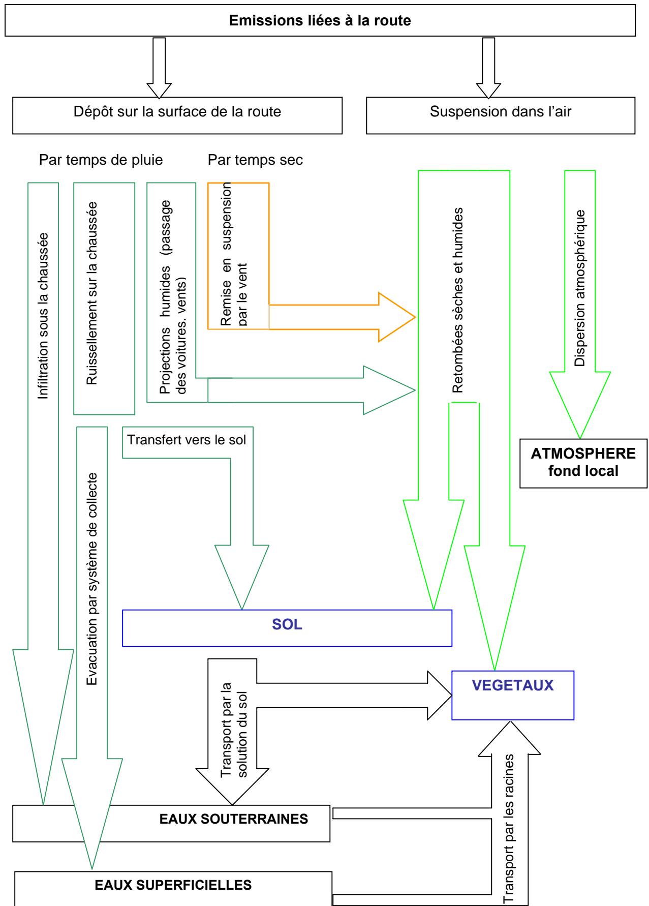
Figure 1 : Principales voies de dispersion des polluants émis en milieu routier (d'après [26])
