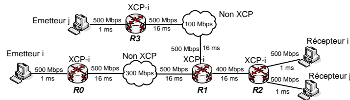
Figure 7: 2 files d'attente non-XCP partageant un chemin XCP
