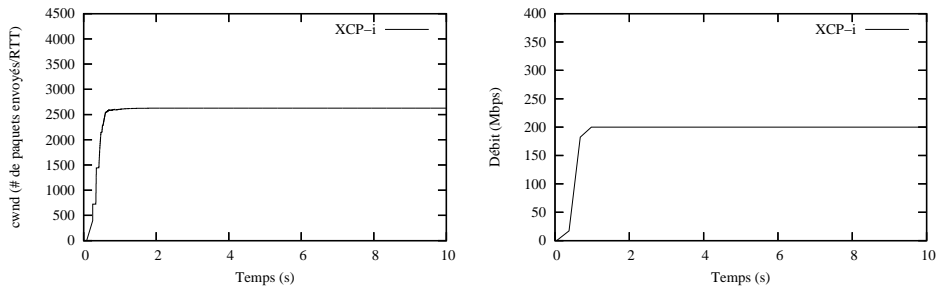
Figure 6: Fenêtre de congestion et débit dans le scénario de déploiement incrémental
