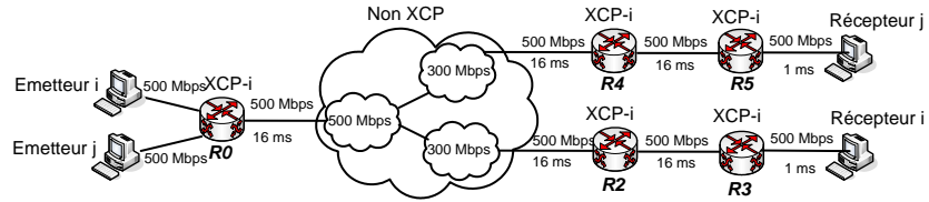
Figure 9: Une file d'attente non-XCP est partagée par des noeuds XCP
