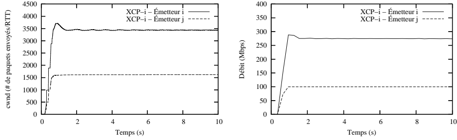
Figure 8: Fenêtre de congestion et débit dans le scénario de Fusion
