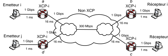
Figure 12: Un goulot d'étranglement partagé par n chemins XCP
