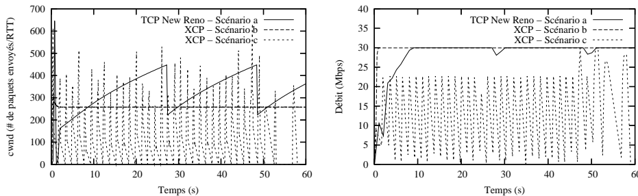
Figure 2: Évolution de la fenêtre de congestion et débit pour les scénarios a,b et c.
