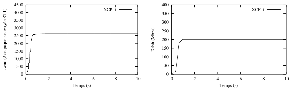
Figure 6: Fenêtre de congestion et débit dans le scénario de déploiement incrémental
