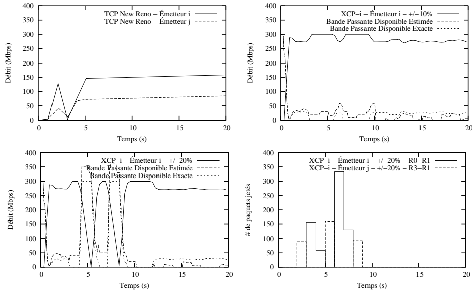
Figure 11: (h.g.) débit pour TCP. (h.d.) XCP-i, Emetteur i, 10%. (b.g) XCP-i, Emetteur i, 20%. (b.d.) pertes de paquets XCP-i, 20%
