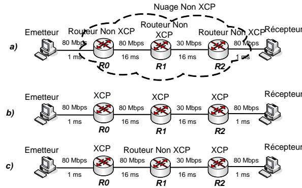
Figure 1: (a) scénario pour TCP, (b) et (c) scénarios pour XCP.
