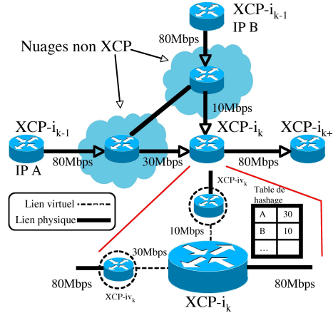
Figure 3: Routeur XCP-i avec un routeur virtuel par nuage non-XCP.
