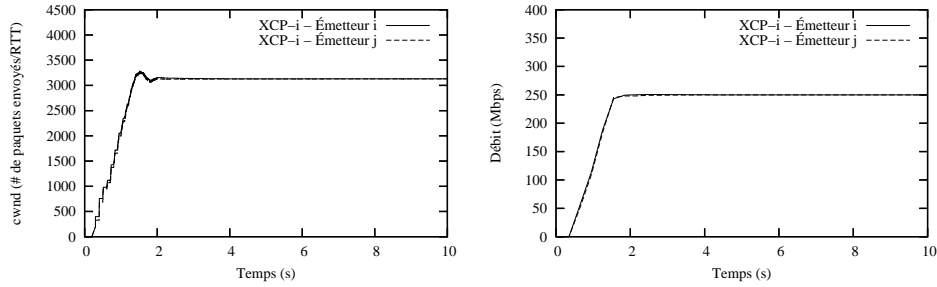
Figure 10: Fenêtre de congestion et débit dans le scénario de duplication
