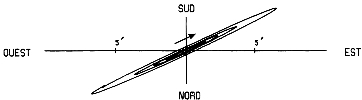
ORBITES APPARENTES
