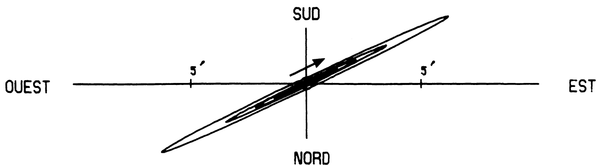
ORBITES APPARENTES
