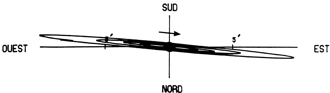
ORBITES APPARENTES
