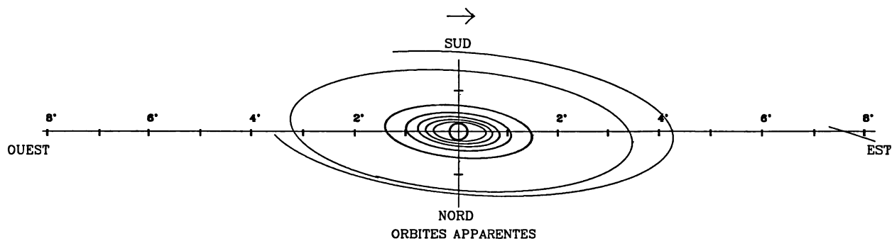
ORBITES APPARENTES
