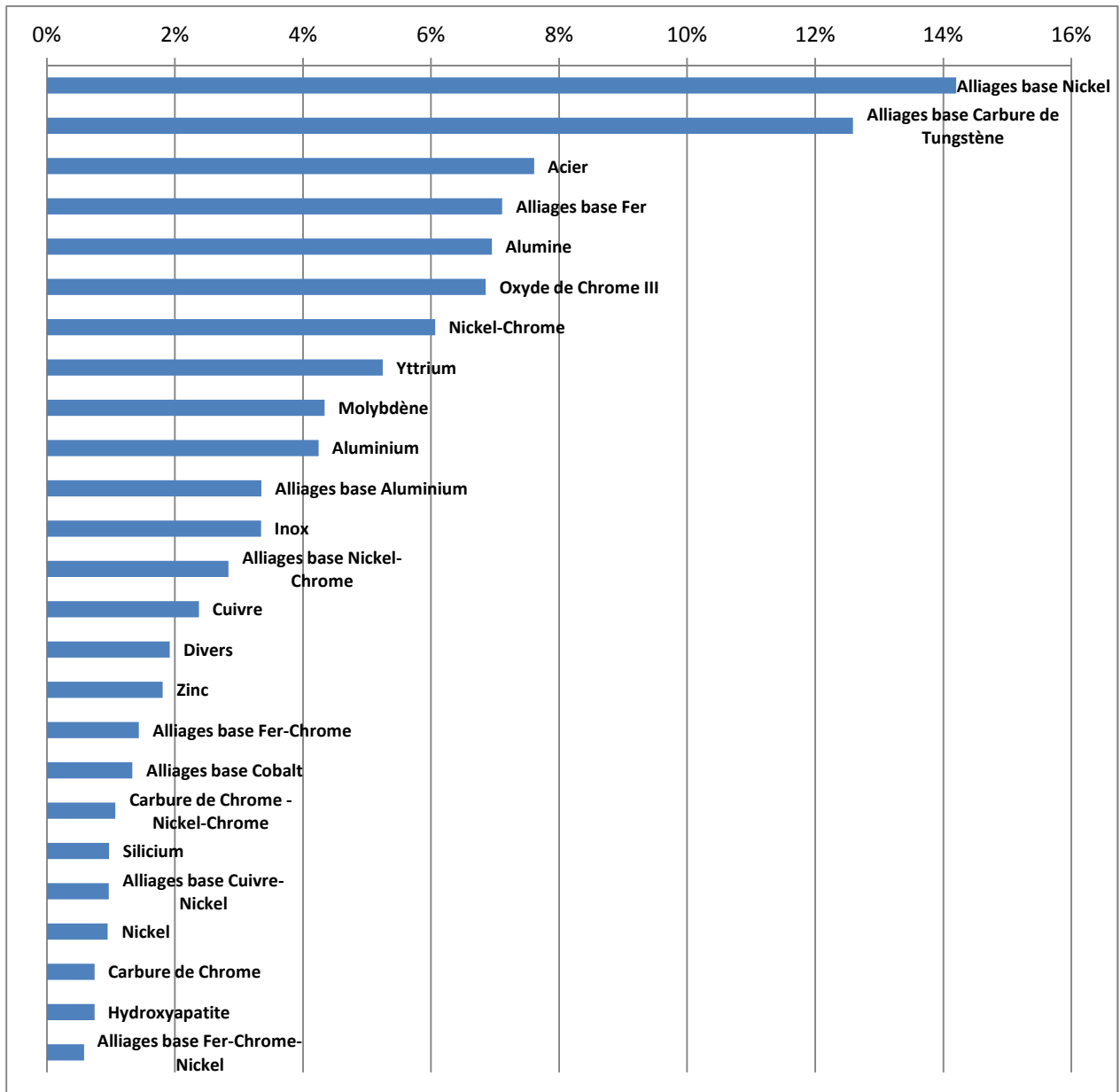
Figure 54 : Répartition des matériaux projetés par le procédé par plasma
