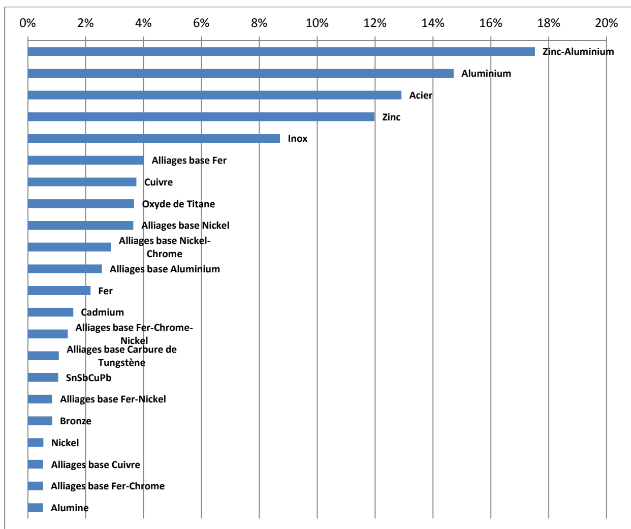
Figure 30 : Répartition des matériaux projetés par le procédé par arc électrique
