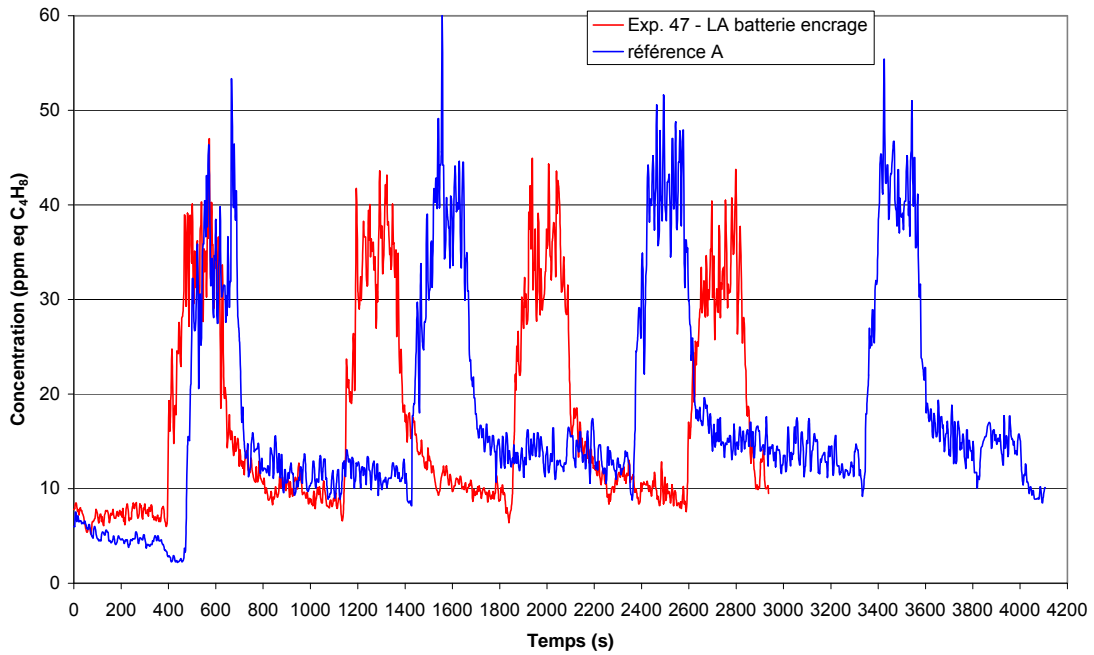
Graphique 39. Influence du lavage automatique de la batterie d'encrage
